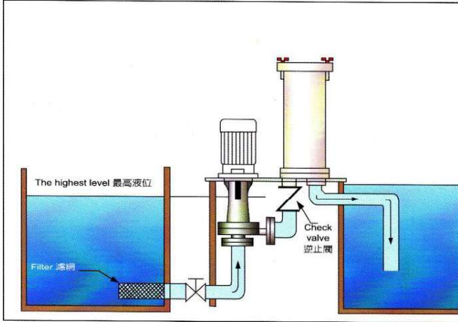
▽ 泵浦裝置桶外，配合過濾器使用 Installed outside tank for filter .
