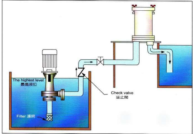
▽ 泵浦裝置桶內，配合過濾器使用 Installed inside tank for filter .
