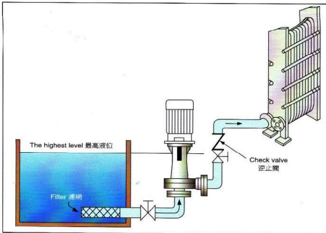
▽ 使用於熱交換器 For heat exchanger.
